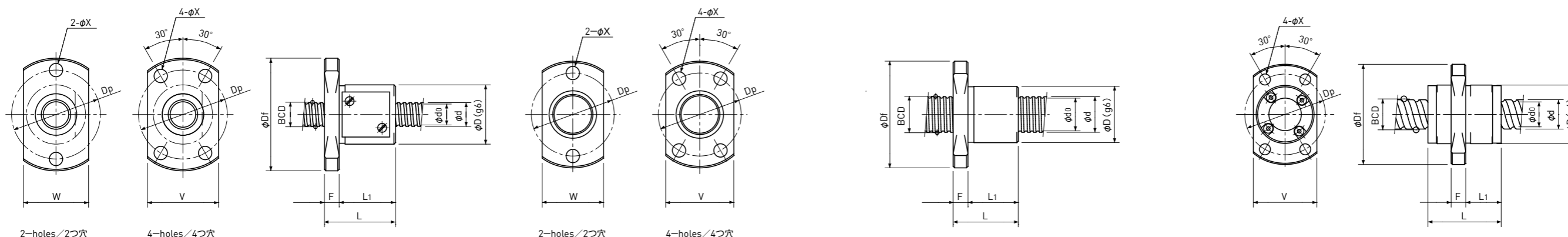
Type-1:Return-plate type リターンプレート式
