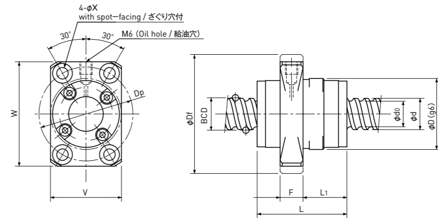
Type-5: End-deflector type エンドデフレクタ式
