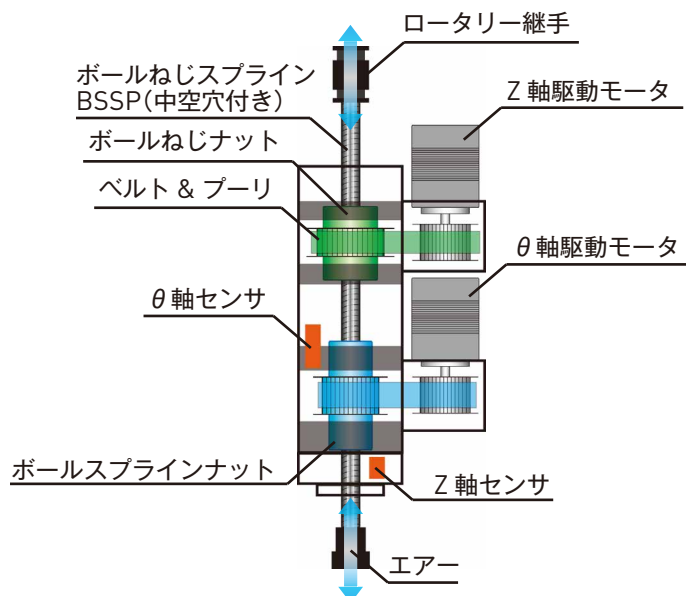
【Belt Drive/ ベルトドライブ】
